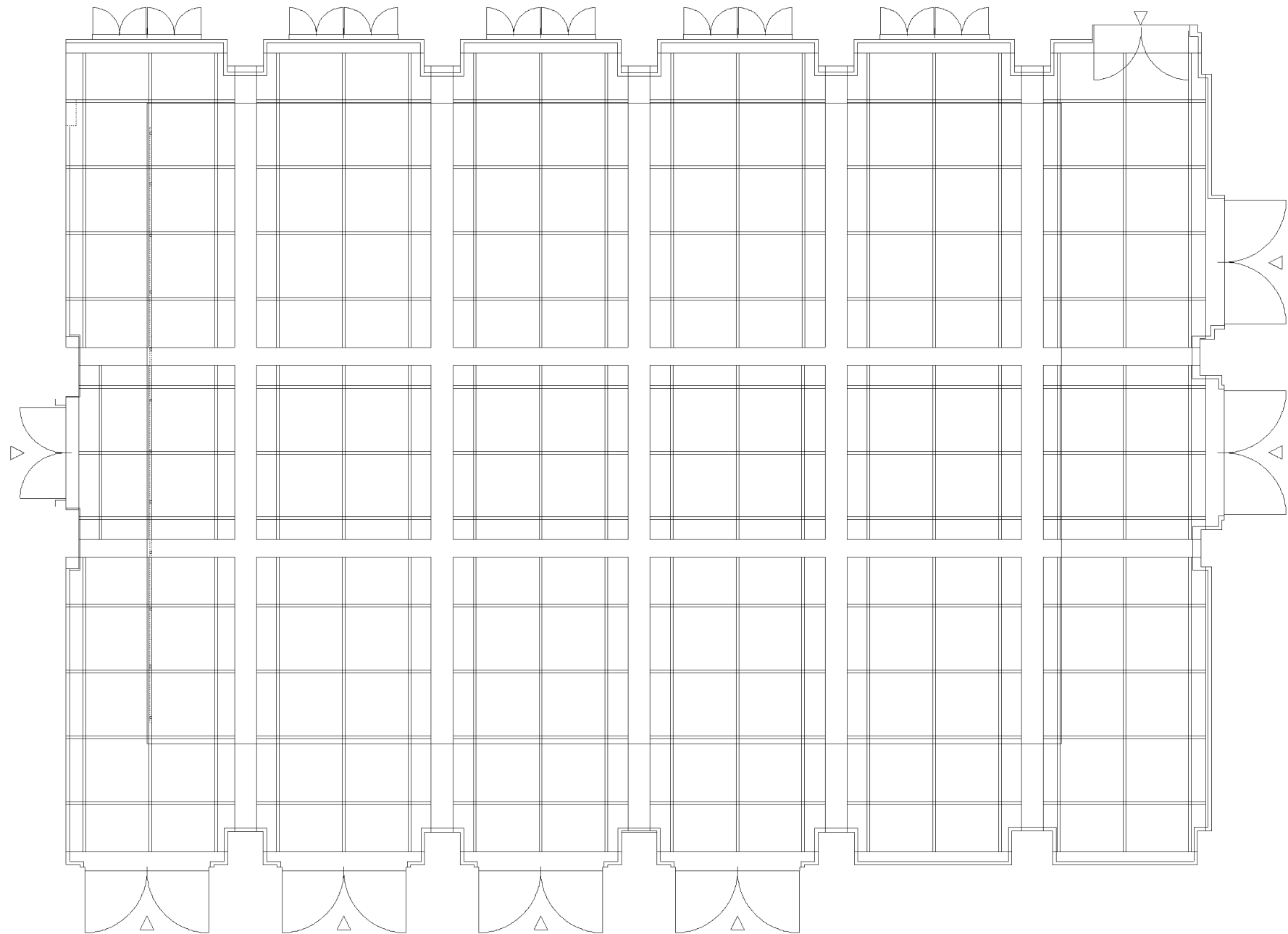
京都芸術センター 1階 フリースペース 天井伏図 1/100
