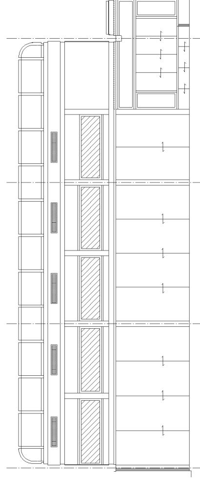
京都芸術センター 2階 大広間 立面図
